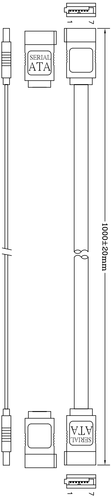
SERIAL ATA 7P(180°) (成型黑色)
